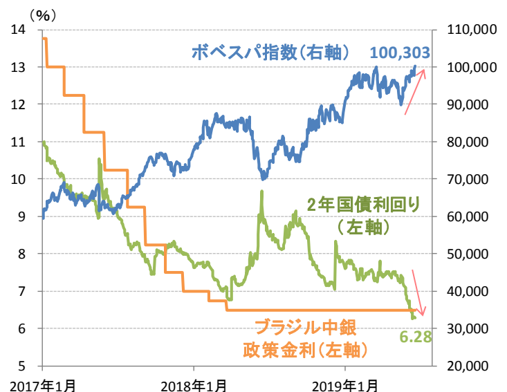
図2：ブラジルのボベスパ指数と2年国債利回り
