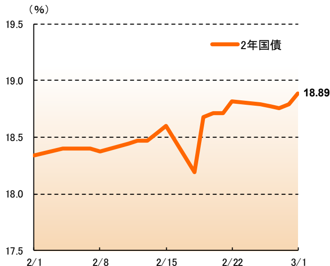
【トルコ 金利推移】 (2019年2月1日～2019年3月1日)
