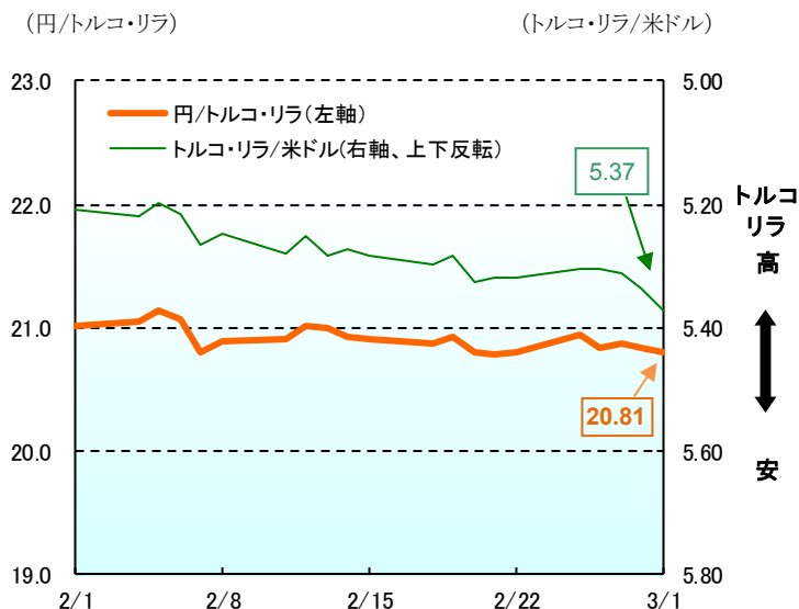
【トルコ・リラ 為替推移】(2019年2月1日～2019年3月1日)
